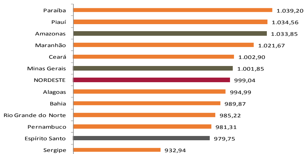
Gráfico 2 - Custo médio da construção civil - Nordeste e os doze estados mais baratos do Brasil - Fevereiro de 2018 (R$/m 2 )
