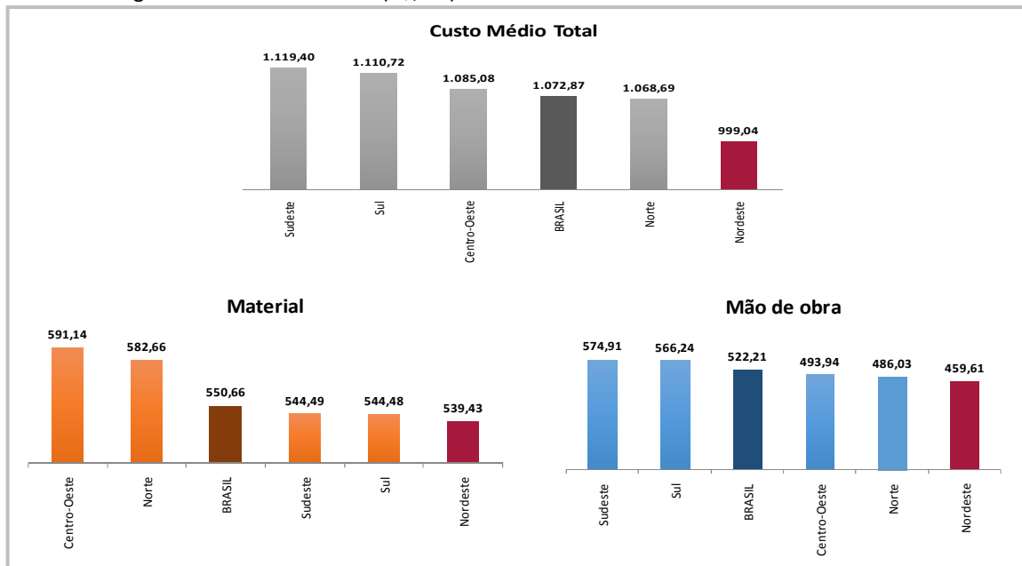
Gráfico 1 - Custo médio total e por componente da construção civil (material e mão de obra) - Brasil e Regiões - Fevereiro de 2018 (R$/m 2 )
