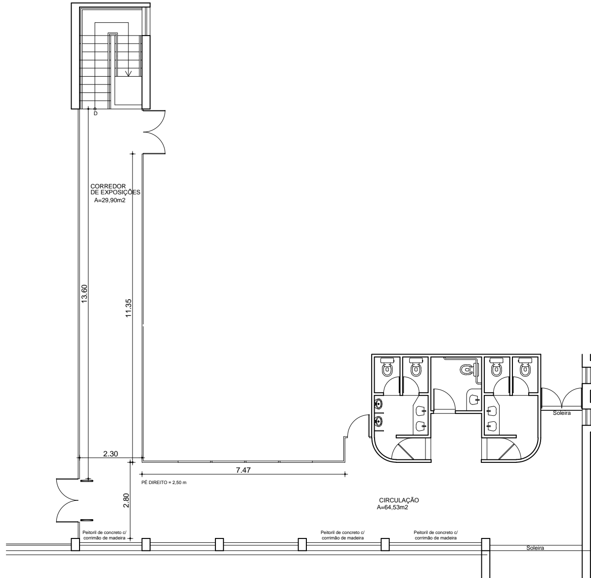
PLANTA PRIMEIRO PAVIMENTO - SOUSA - PB
