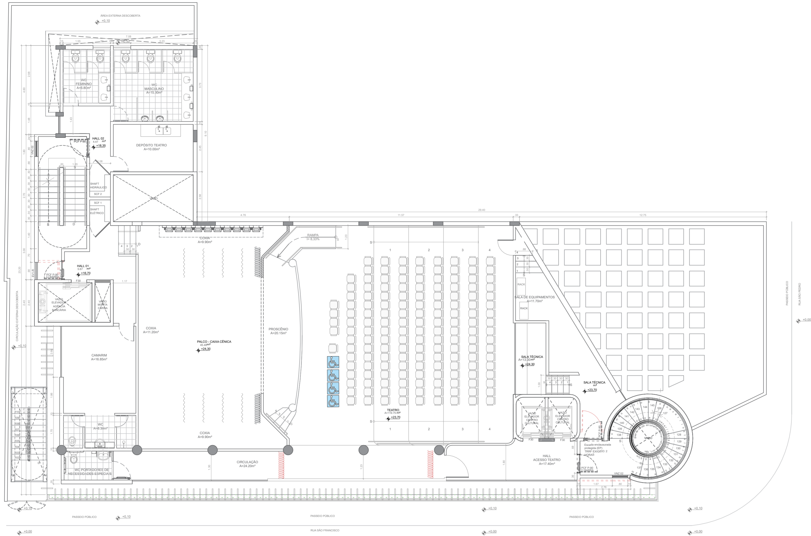
10 PLANTA BAIXA BNB - AGÊNCIA JUAZEIRO DO NORTE -CE 7º PAVIMENTO escala 1/50
