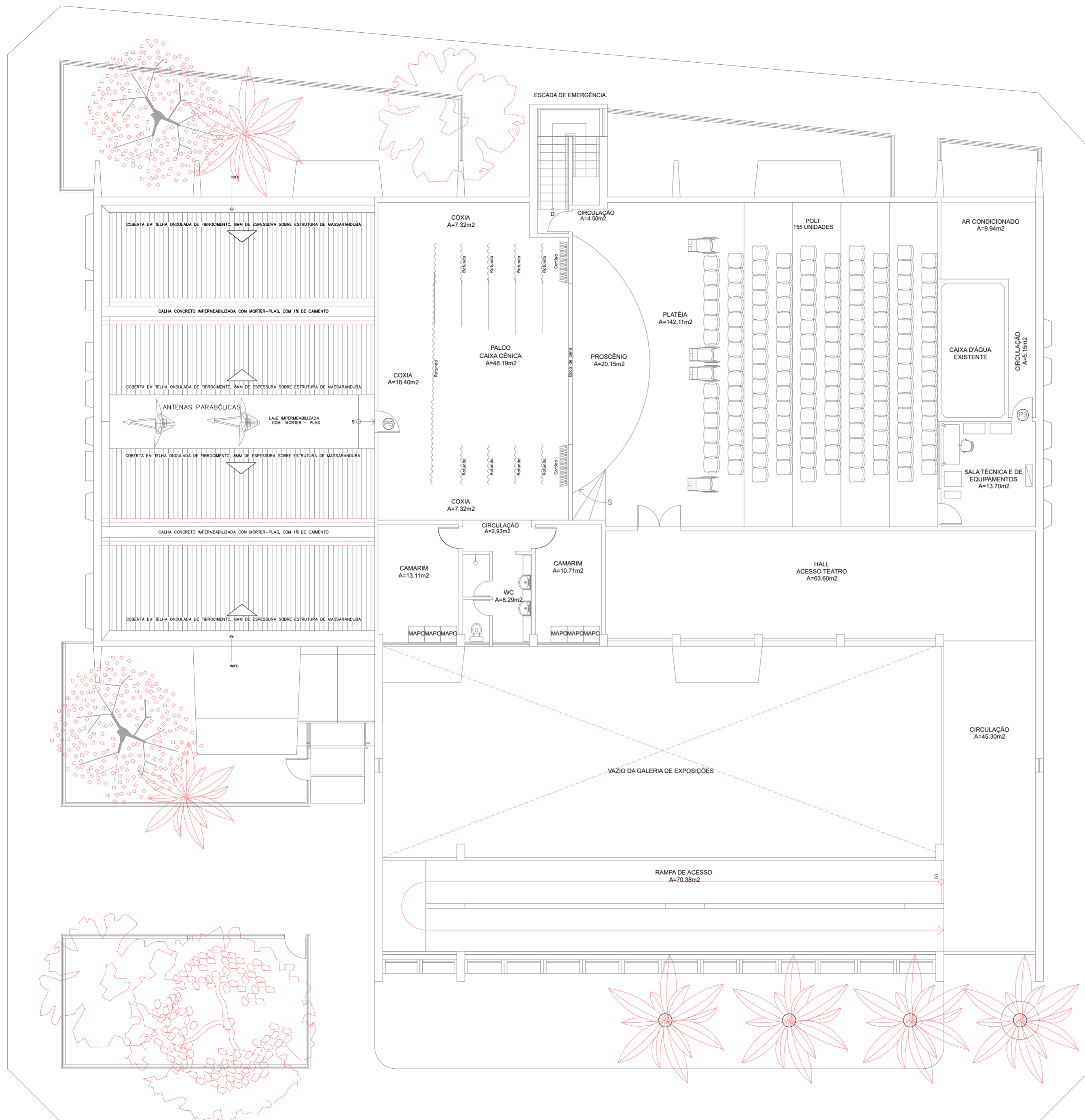
01 PLANTA DE LEIAUTE DO SEGUNDO PAVIMENTO Escala: 1/75
