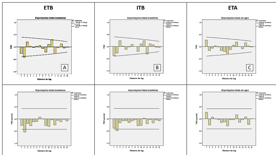
Figura 3 – Correlogramas das Funções de Autocorrelação (FAC) e das Funções de Autocorrelação Parcial (FACP) das séries ETB, ITB e ETA, já diferenciadas
