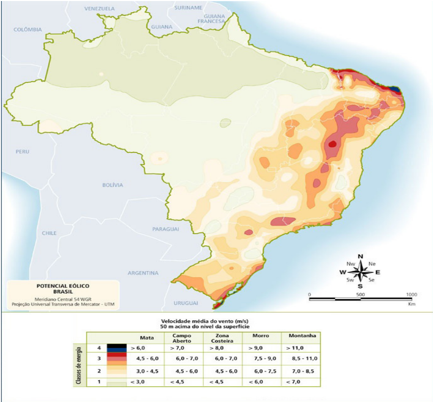
Figura 4 - Velocidade média anual do vento a 50m de altura.
